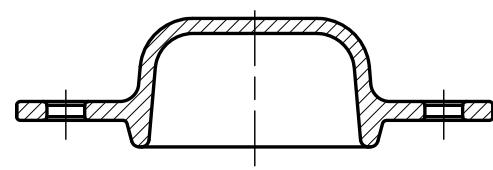
A-A断面
