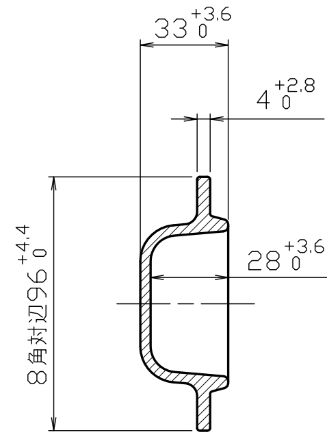
B-B断面
